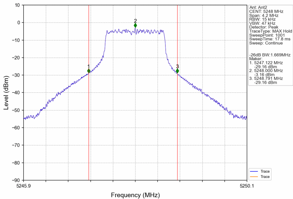
1.4M_HCH_5248MHz_Ant2_NTNV
