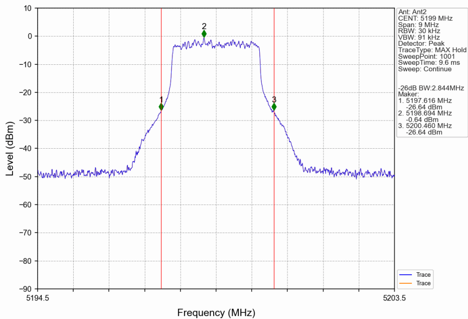
3M_MCH_5199MHz_Ant2_NTNV
