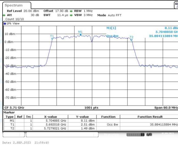
11N40MIMO_Ant2_5710
