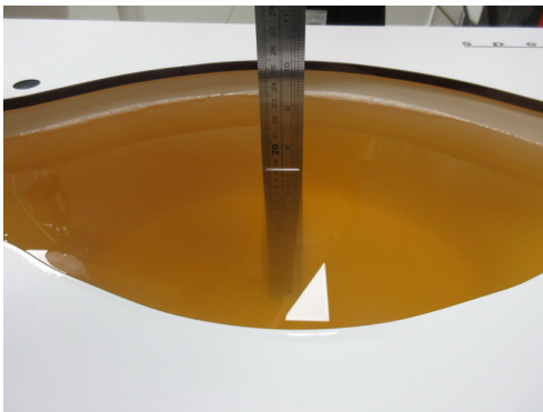
HSL_5GHz_Body_17.5cm
