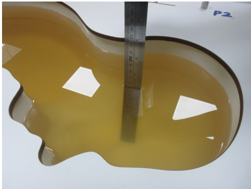
HSL_810MHz-920MHz_Head_15.6cm
