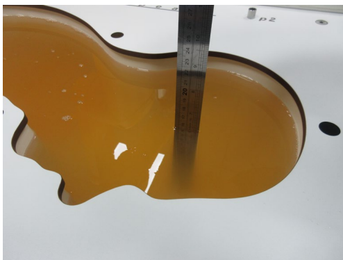
HSL_1700MHz-1900MHz_Head_15.5cm HSL_1700MHz-1900MHz_Body_16.2cm
