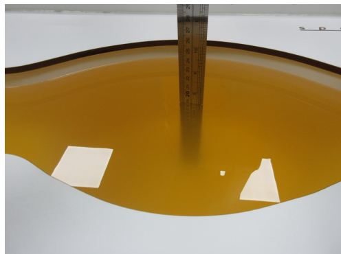
HSL_1900MHz-2300MHz_Head_15.5cm HSL_1900MHz-2300MHz_Body_18.8cm
