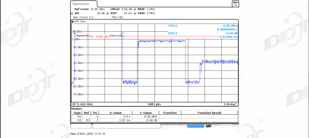
3DH5_Right side_Hop
