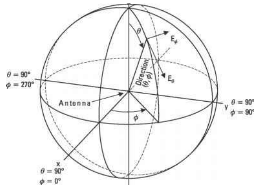
Antenna Coordinates
