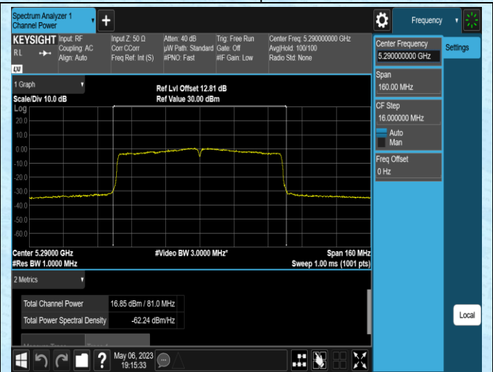
11AC80SISO-Ant2-5290
