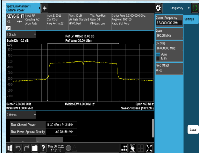
11AC80SISO-Ant1-5530
