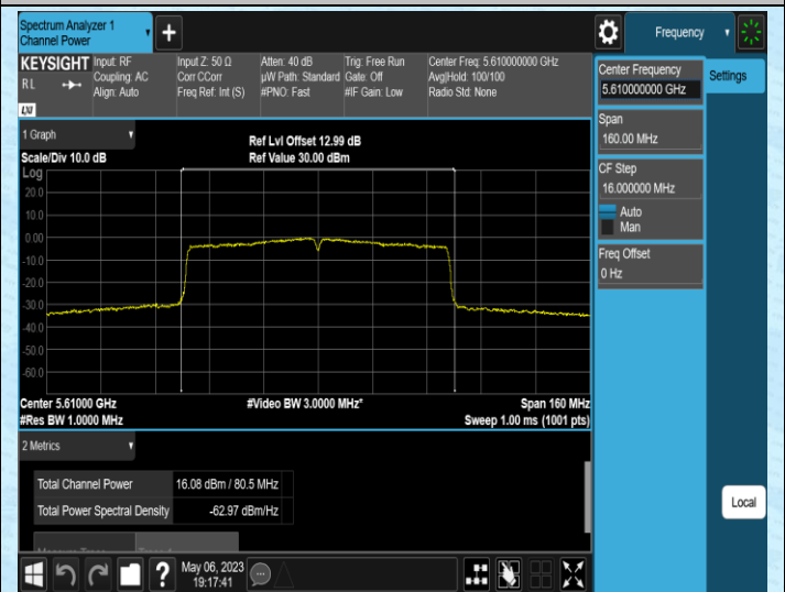
11AC80SISO-Ant2-5610
