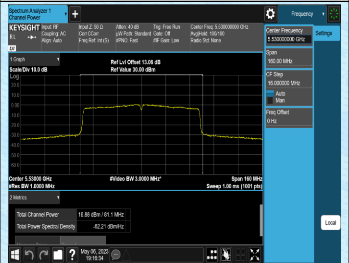
11AC80SISO-Ant2-5530
