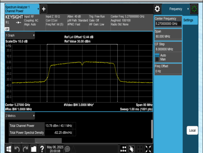
11N40MIMO-Ant2-5270
