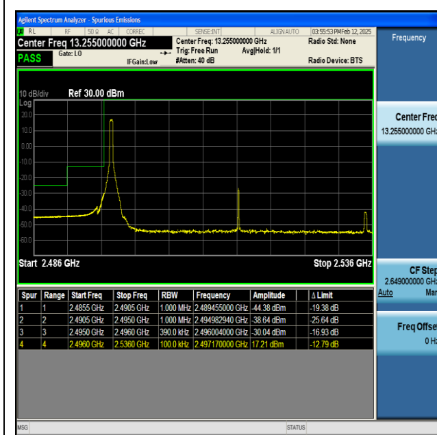
NTNV-n41-PC2-30-40-L-CP-QPSK-Edge_1RB_Left-PASS
