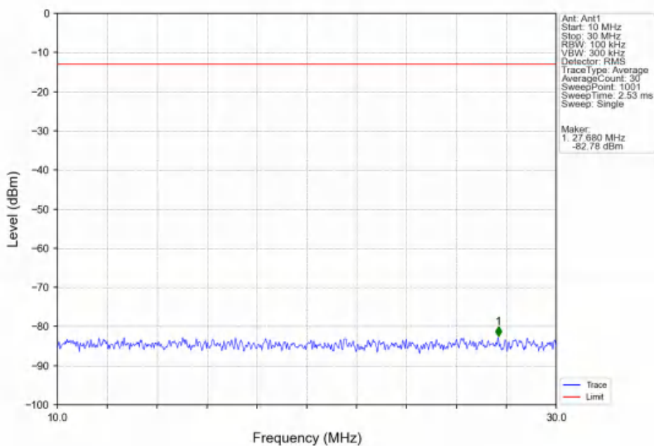
Band66 15MHz QPSK LCH 1717.5MHz RB 1 0 NTV
