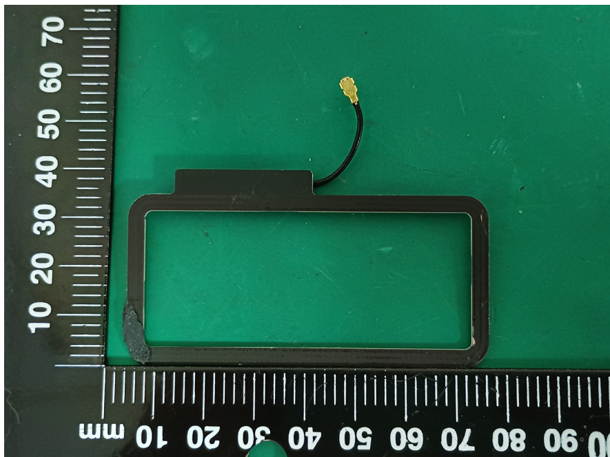
NFC ANT
