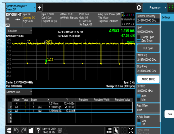
NTNV-11G-Ant1-2437
