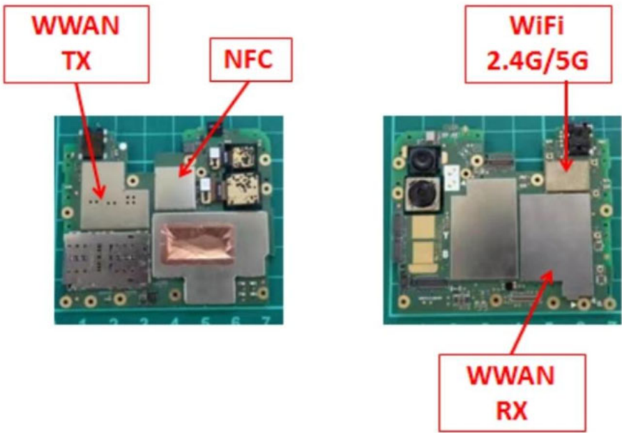
(15) EUT Photo
