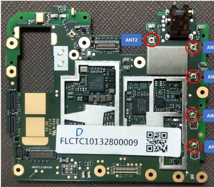
(16) EUT Photo
