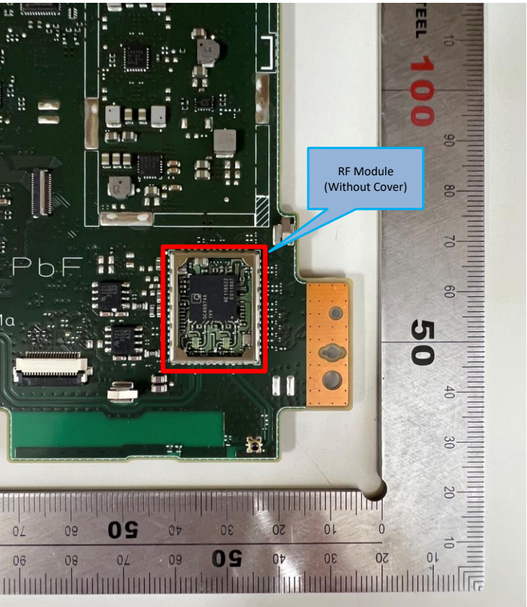
NAVI PCB Back Side 【Figure 4】
