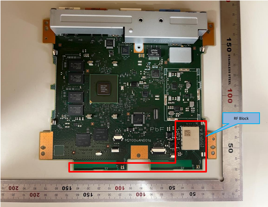
<RF Block Zoom Up> 【Figure 2】
