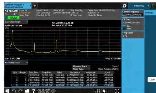
Band41-20MHz-QPSK-41490-1RB#0-PASS
