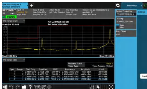
Band41-20MHz-QPSK-39750-1RB#99-PASS
