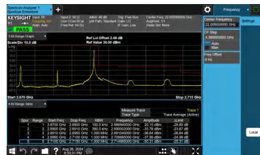
Band41-20MHz-QPSK-41490-1RB#99-PASS
