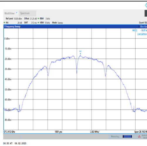
11B-Ant1-2412--16.11-0.04-0.00-0.00
