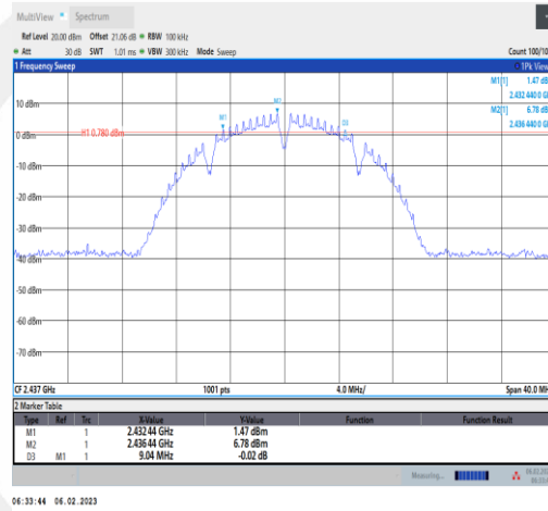
11B-Ant1-2437
