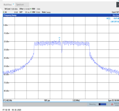
11G-Ant1-2462--19.13-0.26-0.00-0.00
