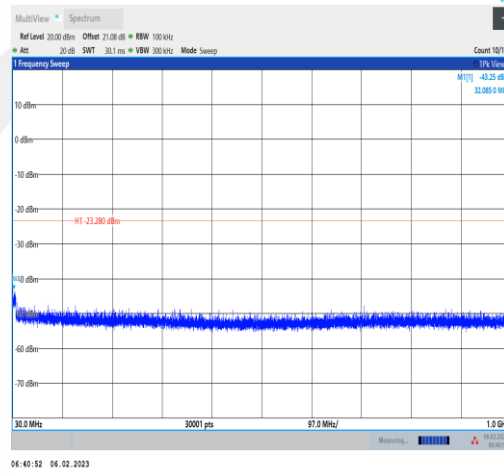
11B-Ant1-2462-30~1000-6.72
