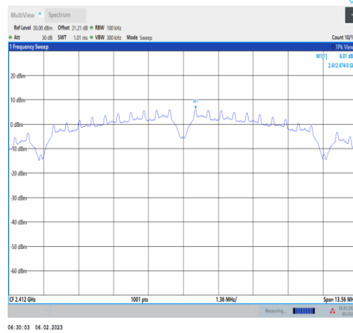
11B-Ant1-2412-2412.47
