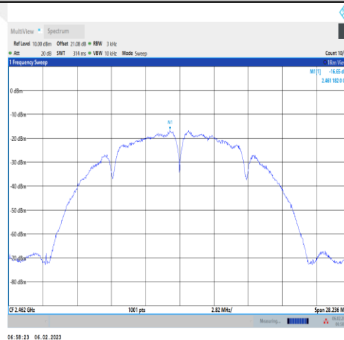
11B-Ant1-2462--16.65-0.00-0.00-0.00
