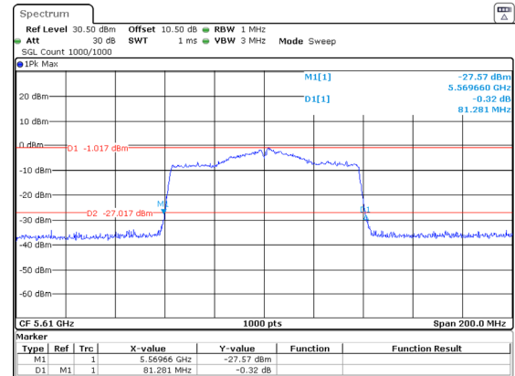
802.11ac80_5610MHz_Chain 1
