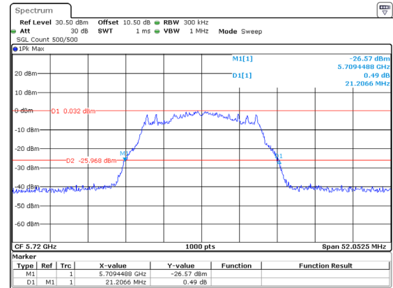
802.11a_5720MHz_Chain 2
