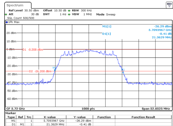
802.11ac20_5720MHz_Chain 2
