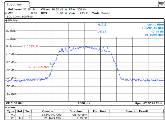
802.11ac20_5580MHz_Chain 2
