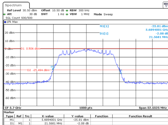
802.11ac20_5700MHz_Chain 2
