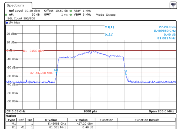
802.11ac80_5530MHz_Chain 2
