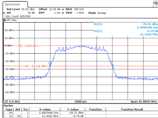
802.11ac20_5500MHz_Chain 2
