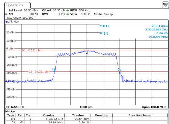
802.11ac40_5550MHz_Chain 2
