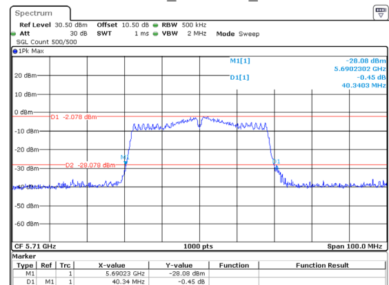
802.11ac40_5710MHz_Chain 2
