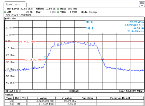
802.11ac20_5580MHz_Chain 1
