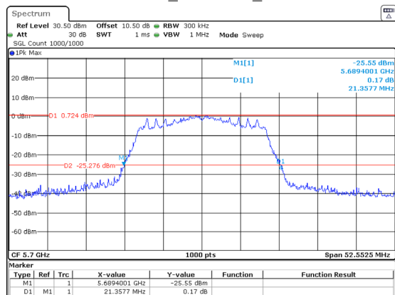
802.11ac20_5700MHz_Chain 1
