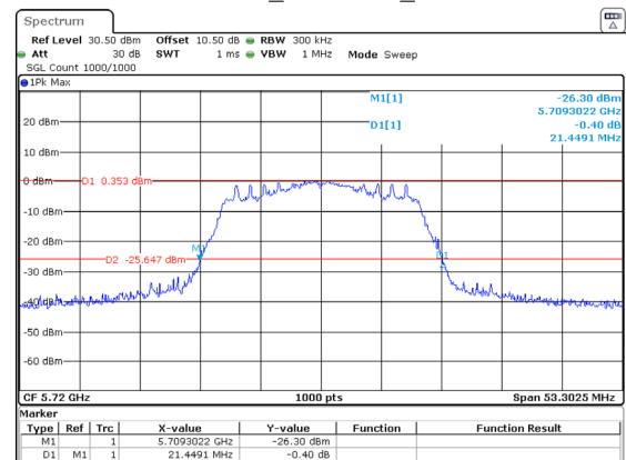
802.11ac20_5720MHz_Chain 1
