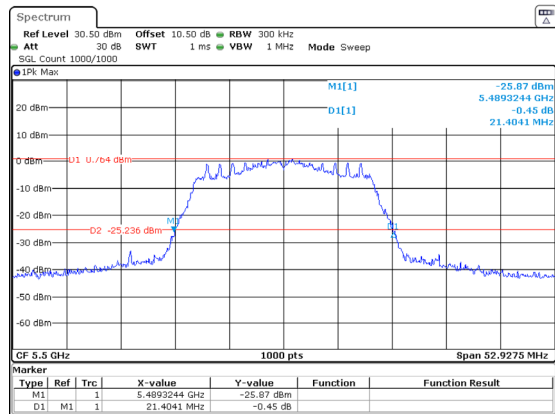
802.11ac20_5500MHz_Chain 1
