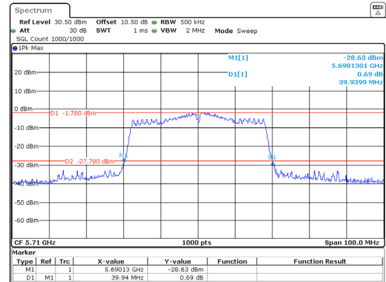
802.11ac40_5710MHz_Chain 1
