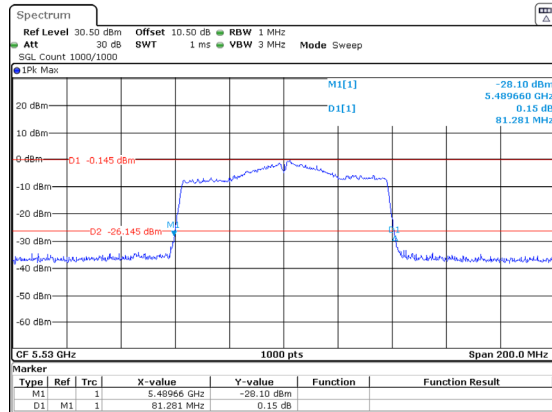
802.11ac80_5530MHz_Chain 1
