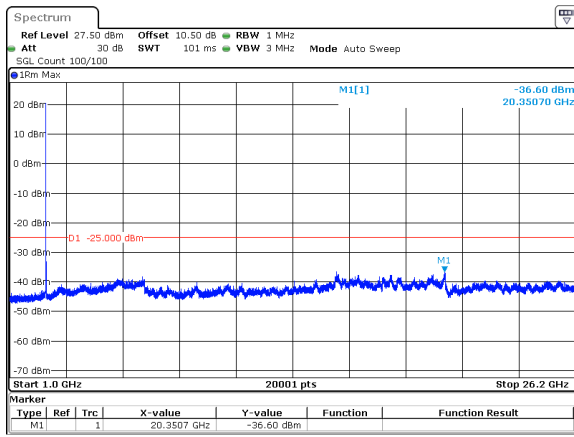
25MHz_30kHz_2607.5MHz_DFT-s-OFDM QPSK_RB1@0&amp;-36.60 dBm
