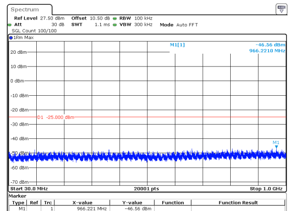
30MHz_30kHz_2585MHz_DFT-s-OFDM QPSK_RB75@0&amp;-46.56 dBm
