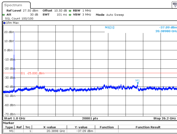
30MHz_30kHz_2595MHz_DFT-s-OFDM QPSK_RB1@0&amp;-37.09 dBm
