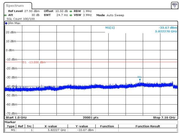
5MHz_15kHz_707.5MHz_DFT-s-OFDM QPSK_RB1@0&amp;-33.67 dBm
