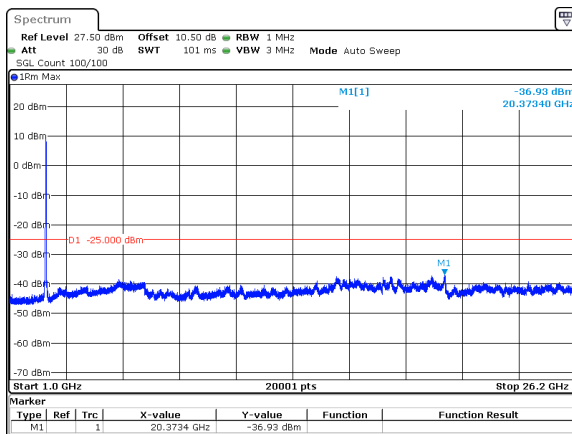
40MHz_30kHz_2600MHz_DFT-s-OFDM QPSK_RB100@0&amp;-36.93 dBm
