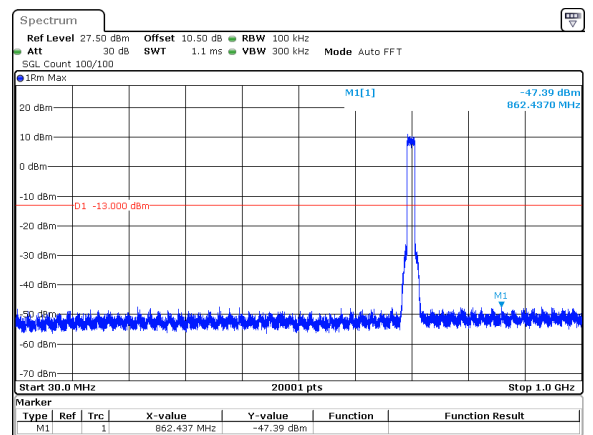
15MHz_15kHz_707.5MHz_DFT-s-OFDM QPSK_RB75@0&amp;-47.39 dBm
