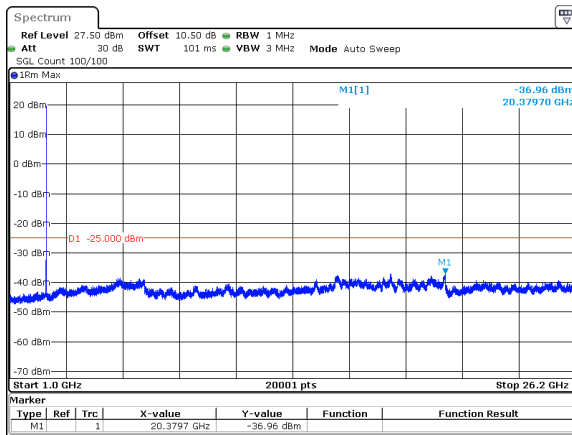
20MHz_30kHz_2610MHz_DFT-s-OFDM QPSK_RB1@50&amp;-36.96 dBm
