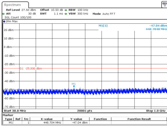
10MHz_15kHz_2685MHz_DFT-s-OFDM QPSK_RB1@0&amp;-47.04 dBm
