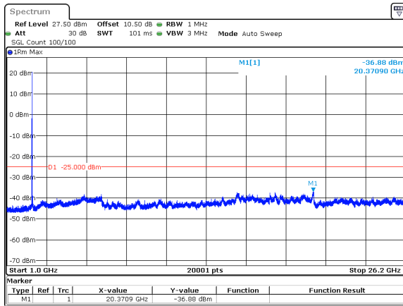
40MHz_30kHz_2600MHz_DFT-s-OFDM QPSK_RB1@0&amp;-36.88 dBm
