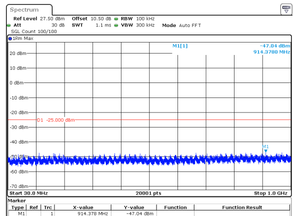
20MHz_30kHz_2580MHz_DFT-s-OFDM QPSK_RB50@0&amp;-47.04 dBm
