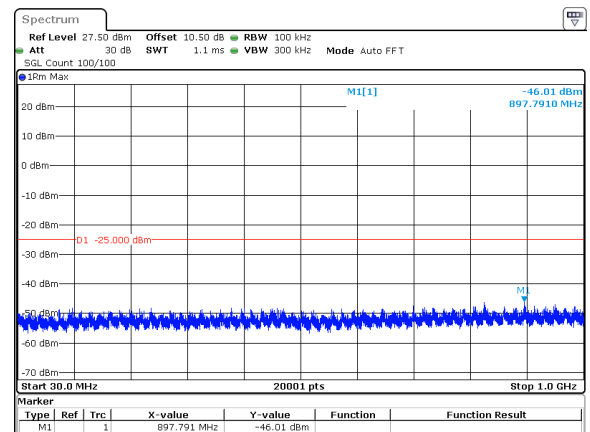
10MHz_30kHz_2595MHz_DFT-s-OFDM QPSK_RB24@0&amp;-46.01 dBm
