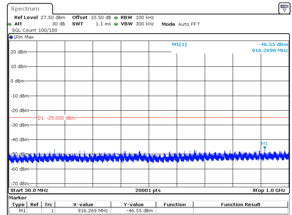
10MHz_15kHz_2685MHz_DFT-s-OFDM QPSK_RB1@51&amp;-46.55 dBm
