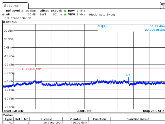
30MHz_30kHz_2585MHz_DFT-s-OFDM QPSK_RB75@0&amp;-36.32 dBm
