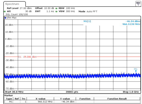
10MHz_30kHz_2595MHz_DFT-s-OFDM QPSK_RB1@0&amp;-46.34 dBm
