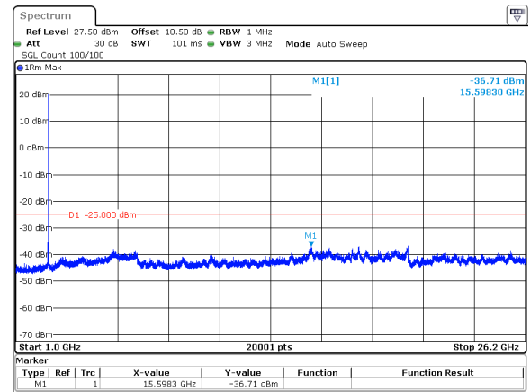
30MHz_30kHz_2585MHz_DFT-s-OFDM QPSK_RB1@77&amp;-36.71 dBm
