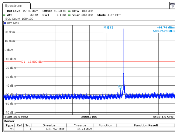
5MHz_15kHz_707.5MHz_DFT-s-OFDM QPSK_RB1@0&amp;-44.74 dBm
