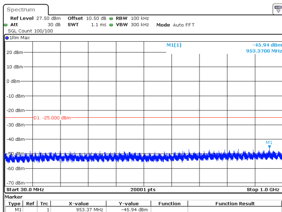
10MHz_30kHz_2615MHz_DFT-s-OFDM QPSK_RB24@0&amp;-45.94 dBm
