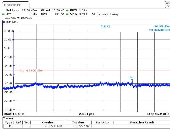
20MHz_30kHz_2580MHz_DFT-s-OFDM QPSK_RB1@0&amp;-36.95 dBm
