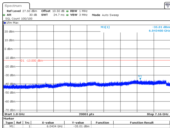
5MHz_15kHz_707.5MHz_DFT-s-OFDM QPSK_RB1@24&amp;-35.01 dBm
