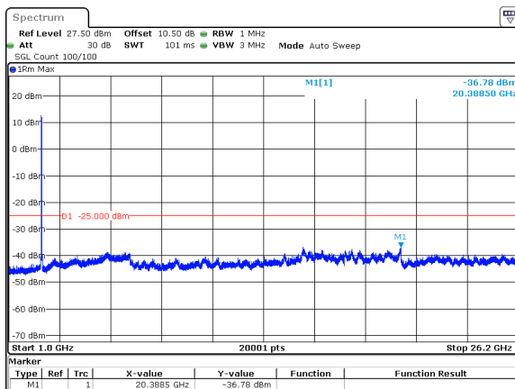
20MHz_30kHz_2610MHz_DFT-s-OFDM QPSK_RB50@0&amp;-36.78 dBm
