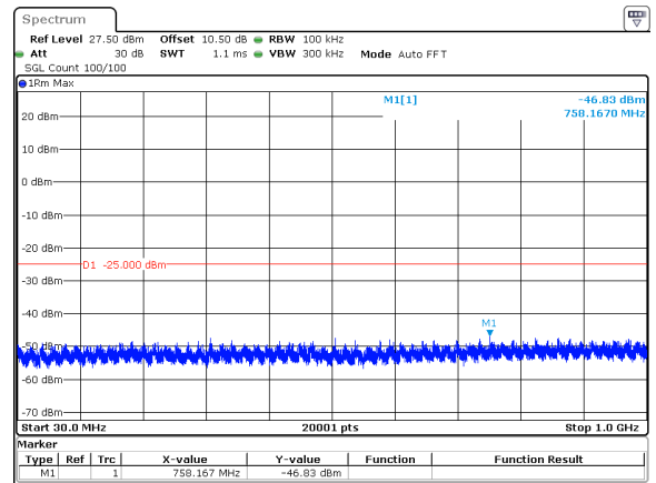
10MHz_30kHz_2615MHz_DFT-s-OFDM QPSK_RB1@23&amp;-46.83 dBm
