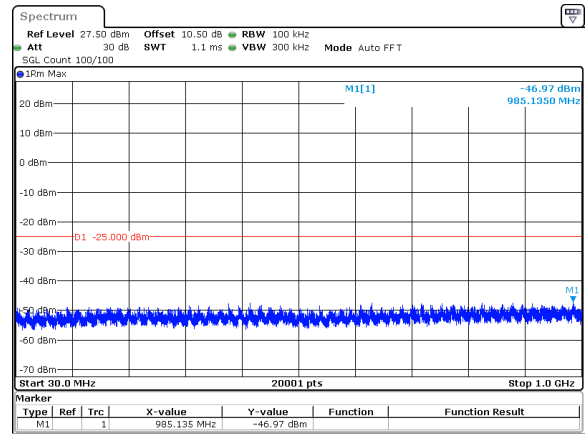
40MHz_30kHz_2590MHz_DFT-s-OFDM QPSK_RB1@0&amp;-46.97 dBm
