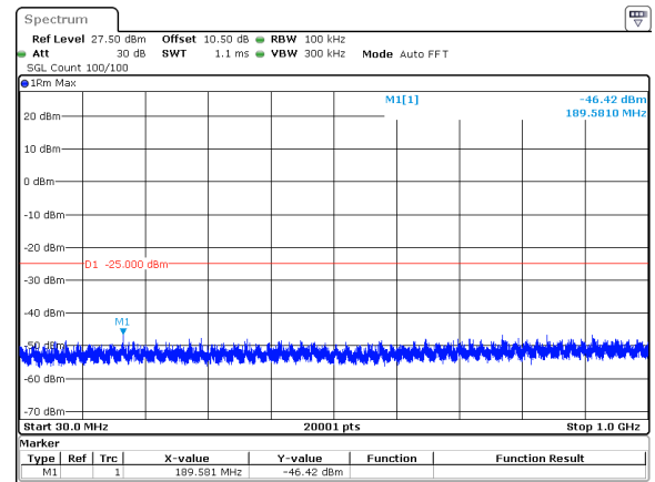
20MHz_30kHz_2610MHz_DFT-s-OFDM QPSK_RB1@50&amp;-46.42 dBm
