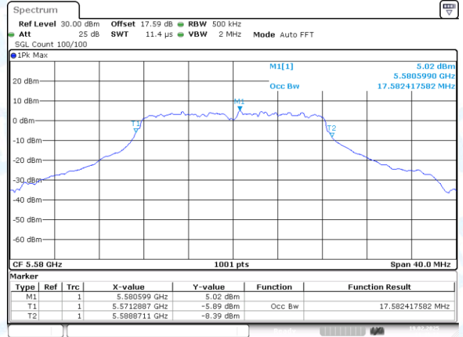
11A-Ant1-5580
