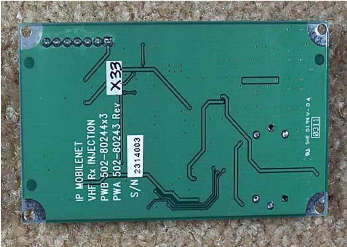
PCB 3 Bottom
