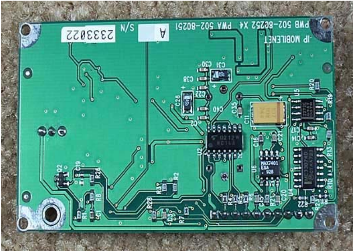
PCB 5 Bottom
