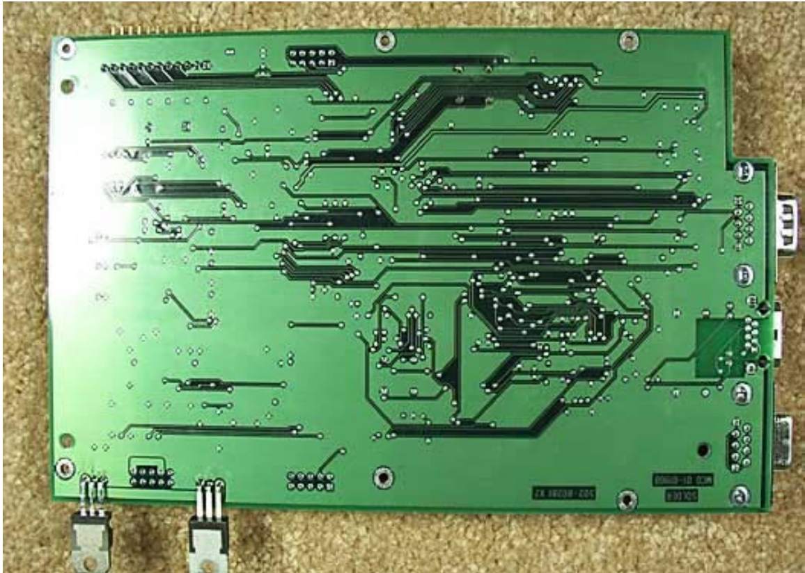
PCB 1 Bottom
