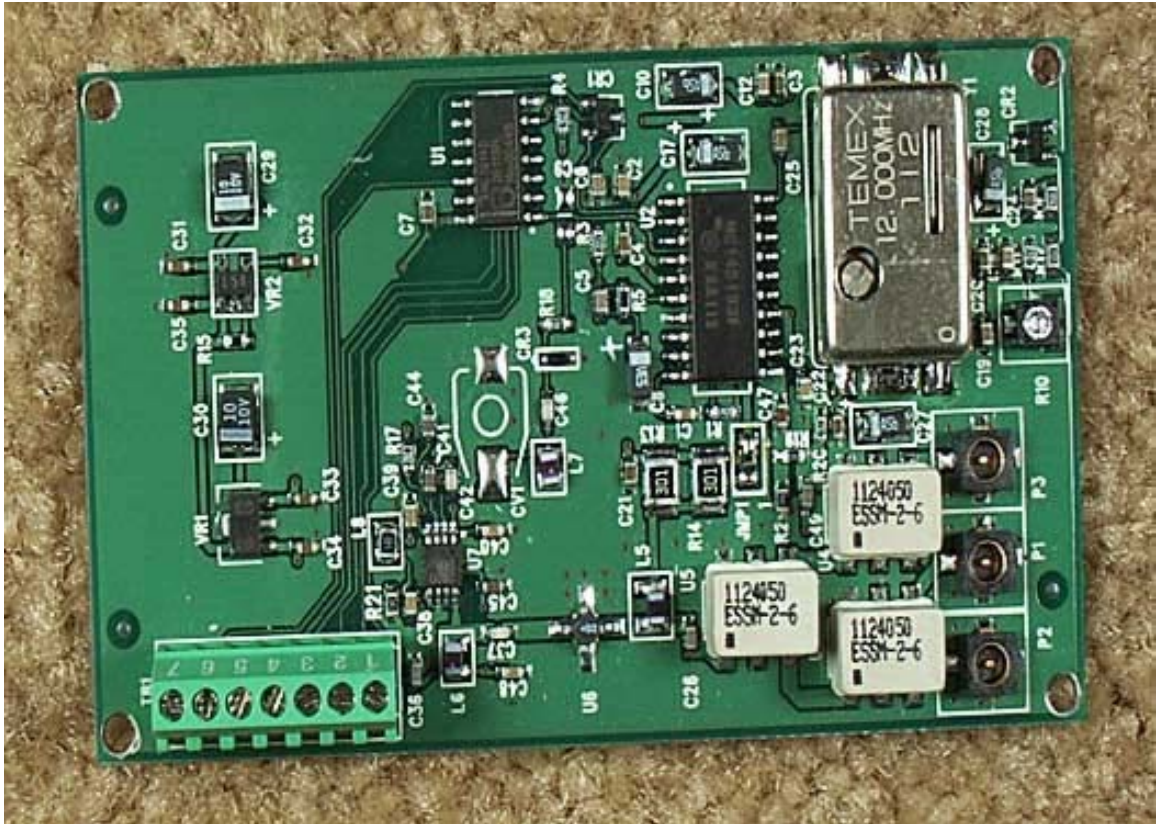
PCB 3 Top
