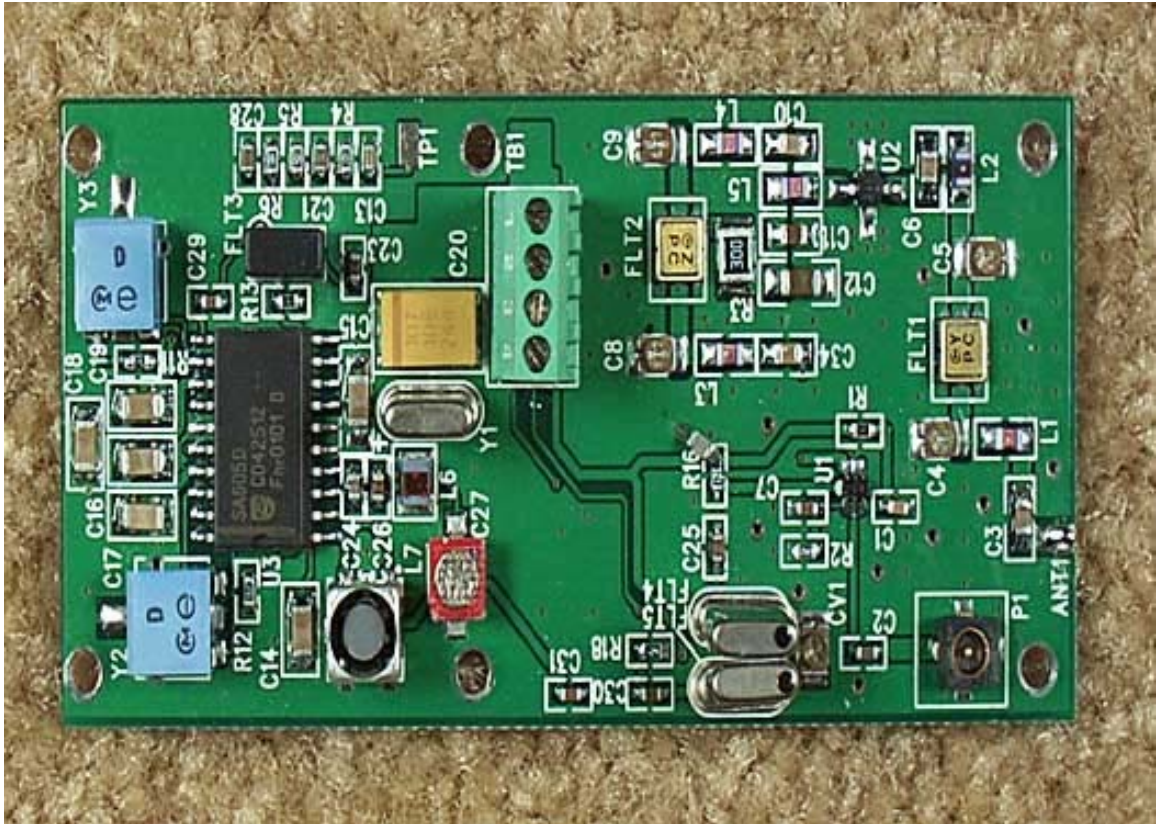
PCB 2 Top
