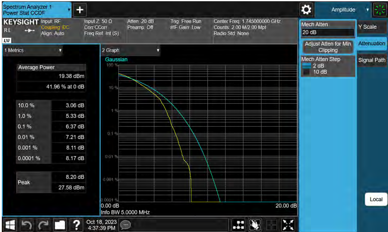
Sub6 n66. PAR Plot (5 M BW_Ch.349000_256QAM_Full RB)
