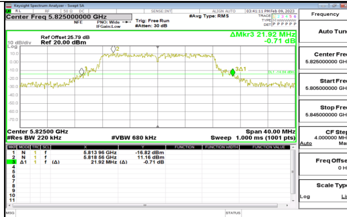
11A-CDD Ant1 5825
