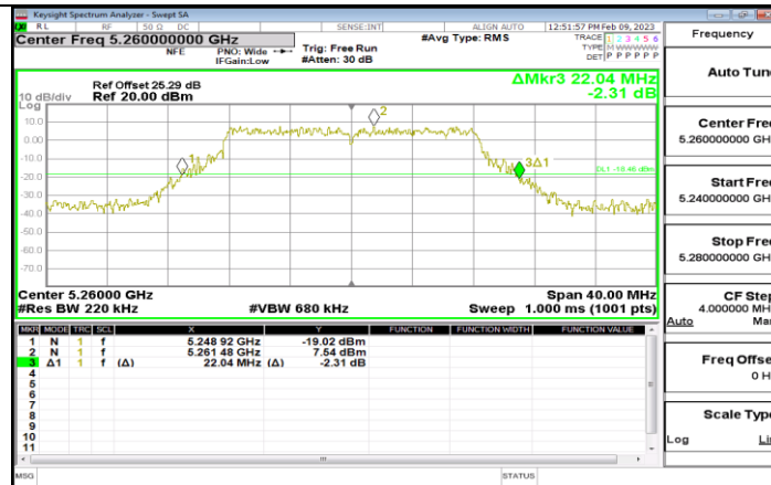
11A-CDD Ant1 5260
