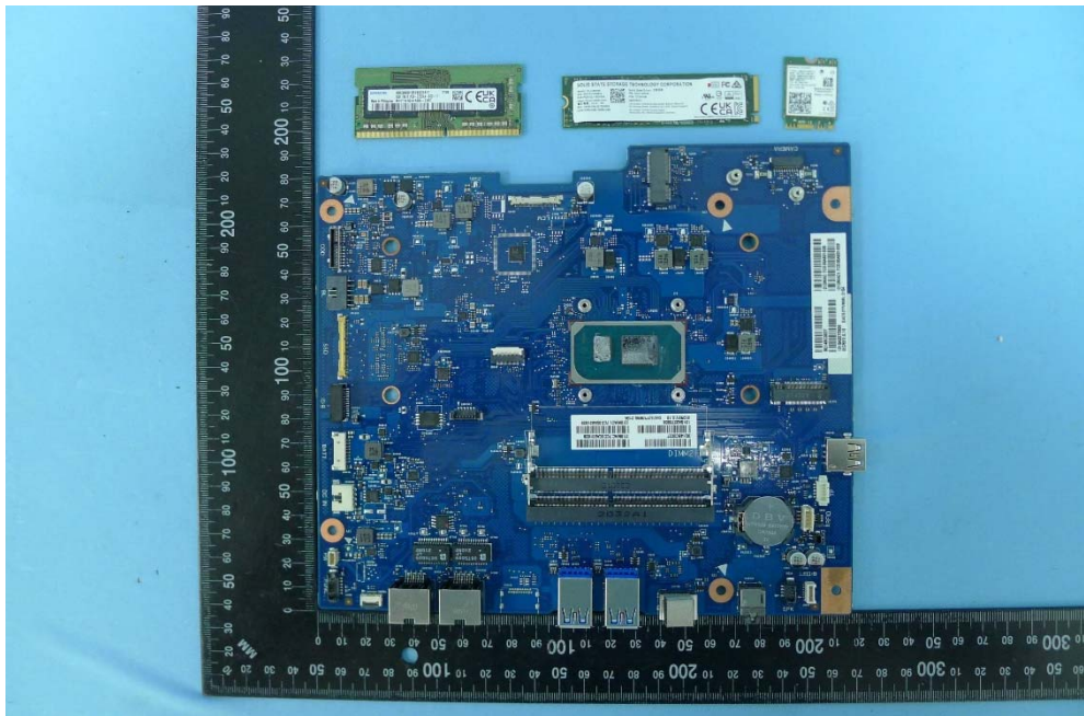
(36) EUT Photo
