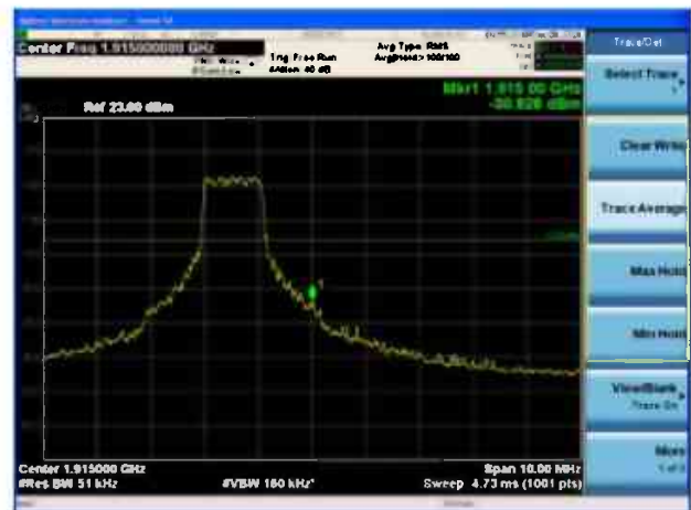
LTE Band 25 20MHz QPSK 1RB CH-High
