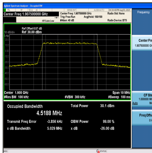
Band2-5MHz-QPSK-19175-25RB#0-4.5188
