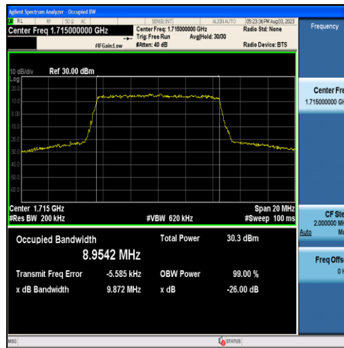
Band4-10MHz-QPSK-20000-50RB#0-8.9542
