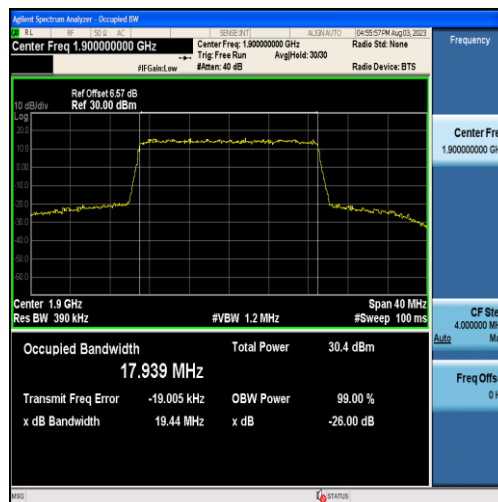
Band2-20MHz-QPSK-19100-100RB#0-17.939
