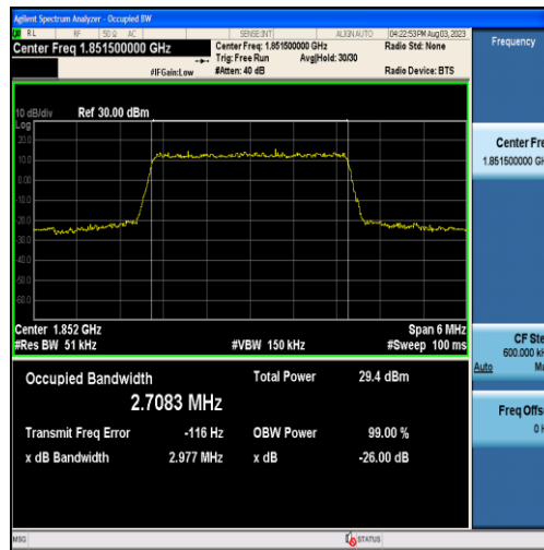
Band2-3MHz-QPSK-18615-15RB#0-2.7083
