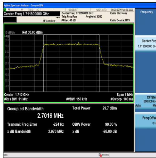
Band4-3MHz-QPSK-19965-15RB#0-2.7016
