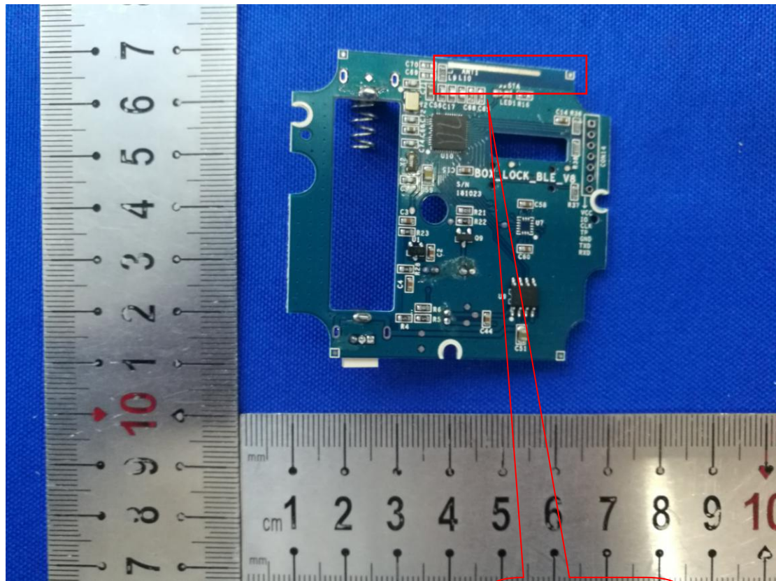
BLE Antenna
