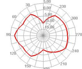
5850.000MHz E2
