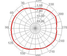
5850.000MHz E2
