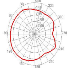
5500.000MHz H
