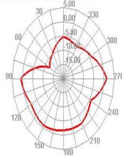
5150.000MHz E1
