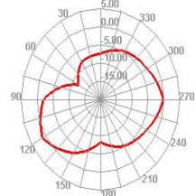
5500.000MHz E1
