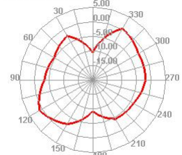
5850.000MHz E1
