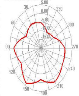
5150.000MHz E2
