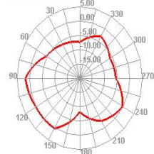
5500.000MHz E2
