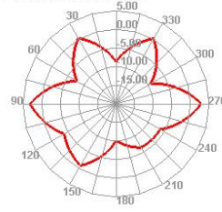
2500.000MHz E1
