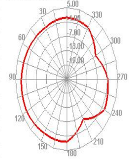
5150.000MHz E2
