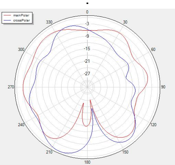
\Phi=90
