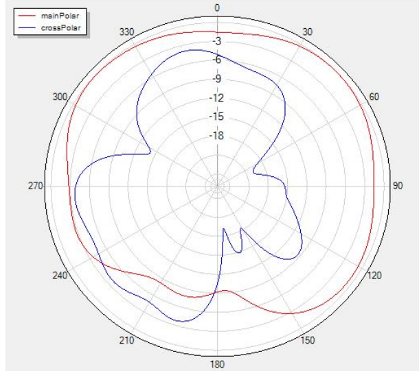
\Phi=0
