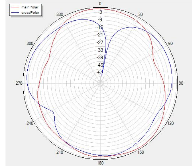
\Theta=90
