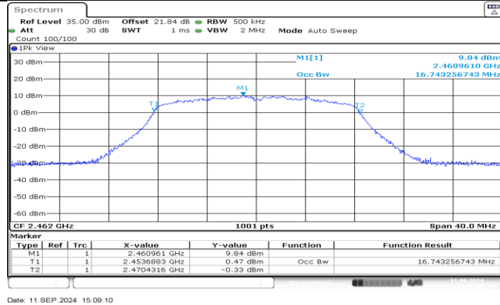
11G_Ant1_2462
