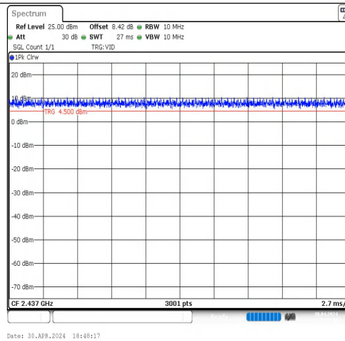
NTNV-11N20MIMO-Ant2-2437
