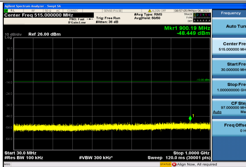
Band2-20MHz-QPSK-19100-1RB#0-30~1000MHz
