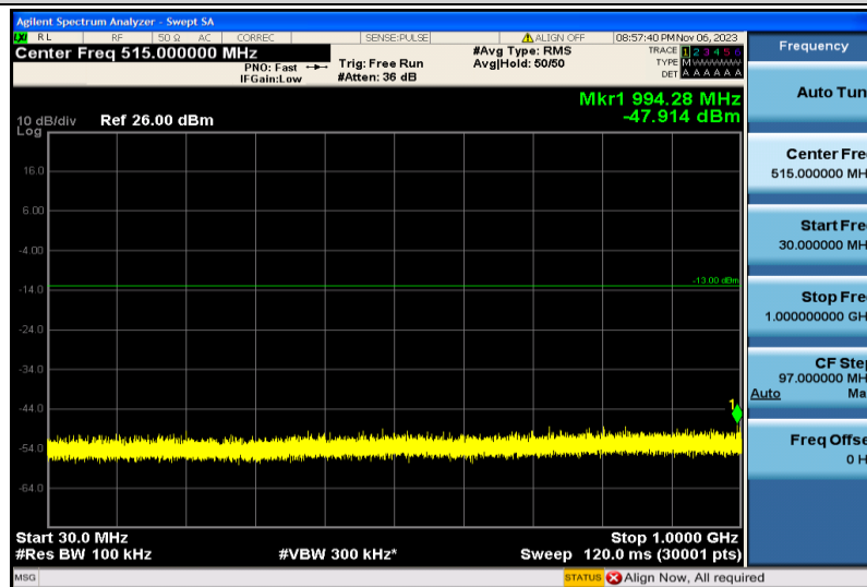
Band2-20MHz-16QAM-19100-1RB#0-30~1000MHz
