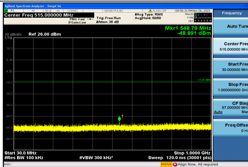
Band4-5MHz-QPSK-20375-1RB#0-30~1000MHz
