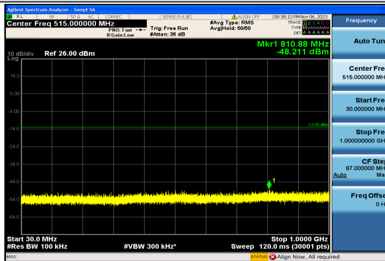
Band4-3MHz-QPSK-20385-1RB#0-30~1000MHz
