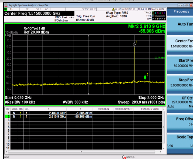
BLE_2402_30~3000
