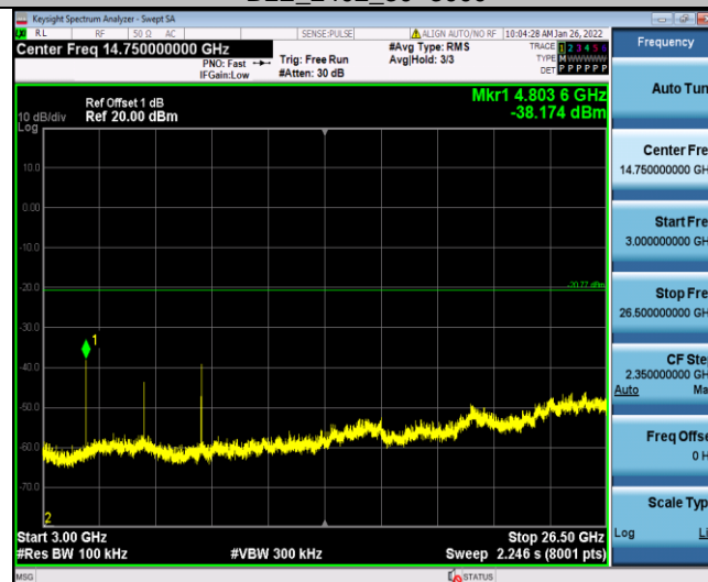
BLE_2402_3000~26500
