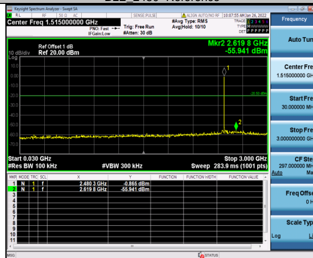
BLE_2480_30-3000
