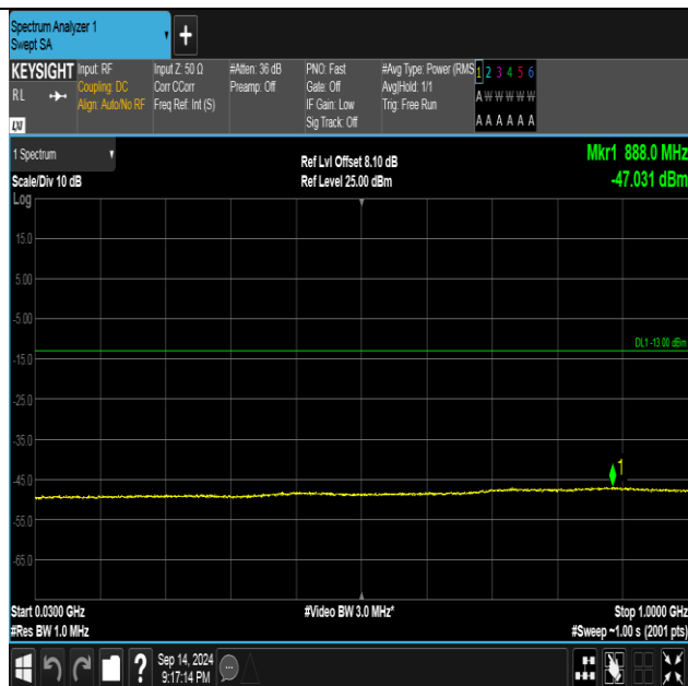
Band2-9538-1-30~1000MHz-PASS
