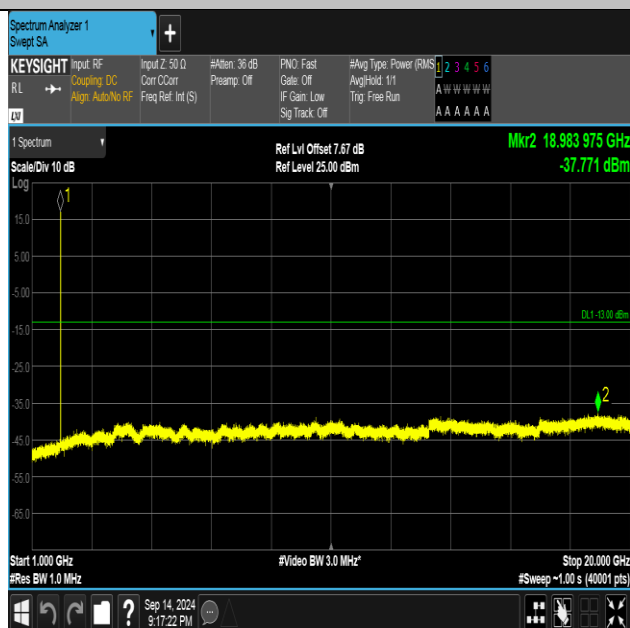
Band2-9538-1-1000~20000MHz-PASS
