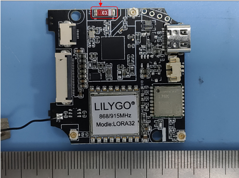
BLE Antenna
