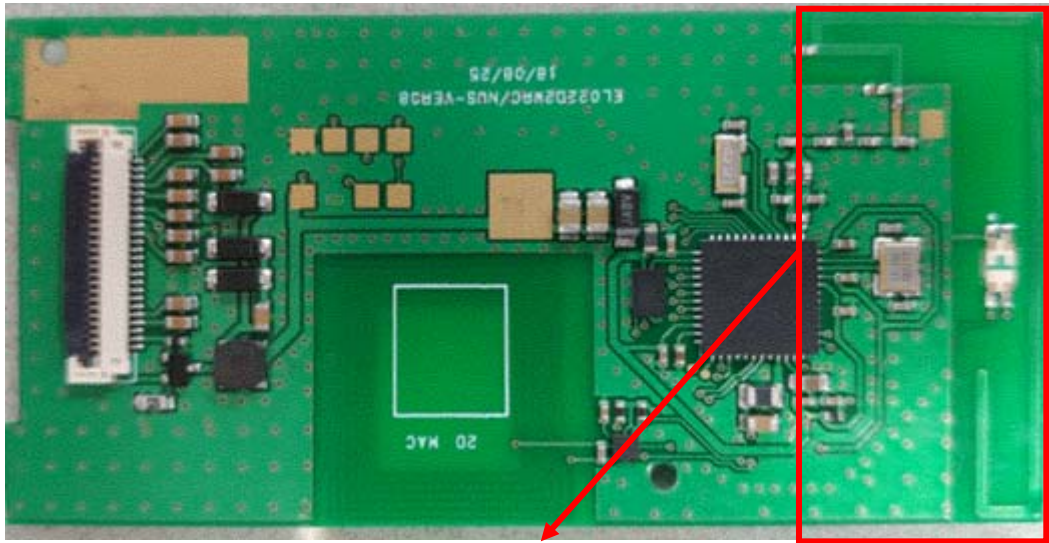
Zigbee Antenna(TX, RX)
