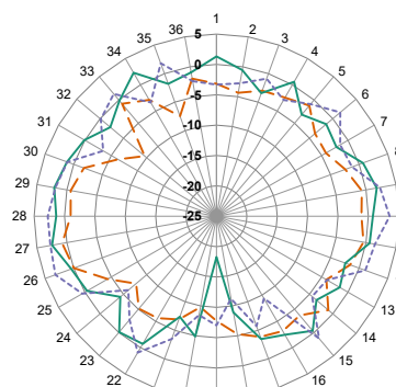
YZ-Plane Gain
