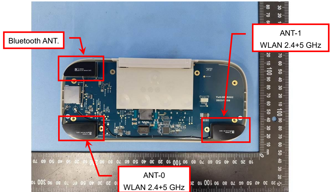
EUT Photo (12)
