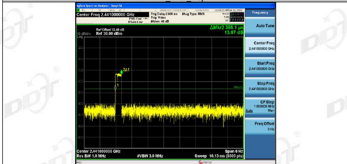
2DH1_Ant1_Hop
