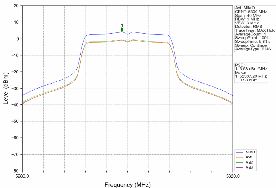
802.11a_MCH_5300MHz_MIMO_NTNV
