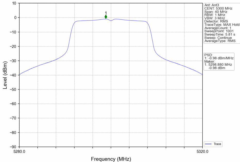
802.11a_MCH_5300MHz_MIMO_NTNV
