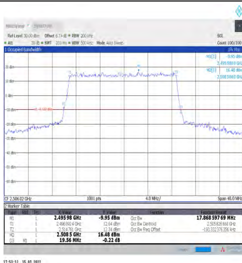
1-N41-30-20-L-1-DFT-QPSK-Outer_Full-50@0-Ant1- 17.869-19.560-≤20-PASS
