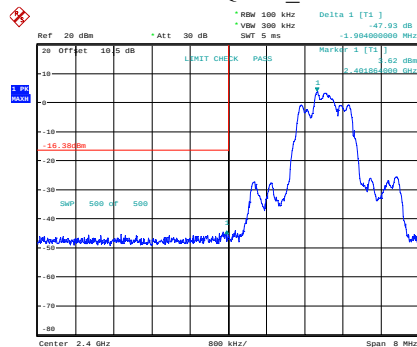
\pi/4 -DQPSK_Low
