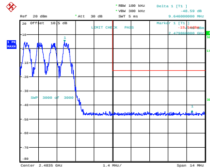
GFSK_Hopping_Upper
