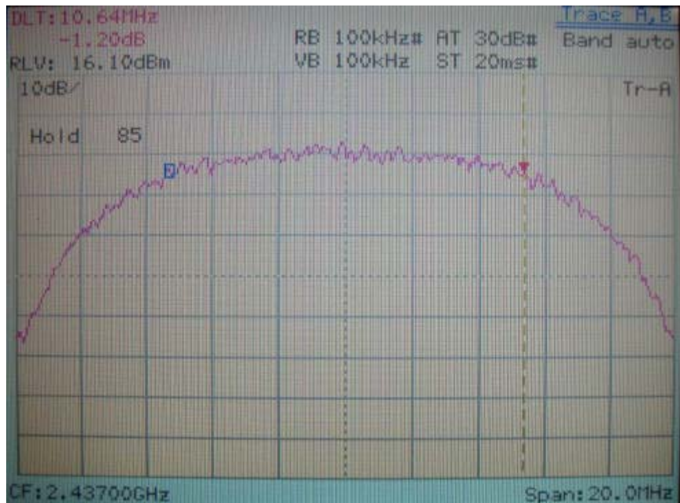
IEEE 802.11b
