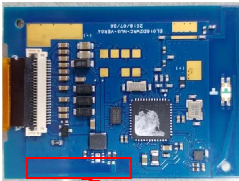
Wake up Antenna(RX)
