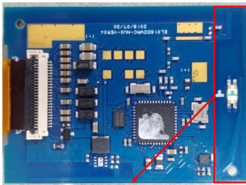
Zigbee Antenna(TX, RX)
