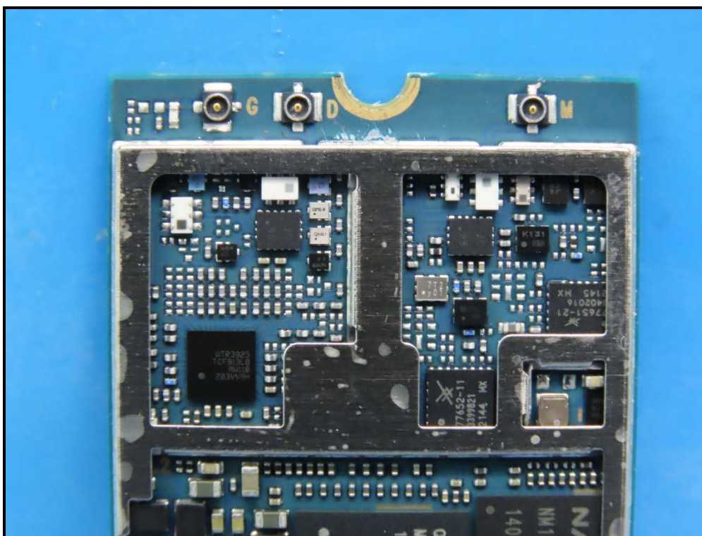
2G ANT
