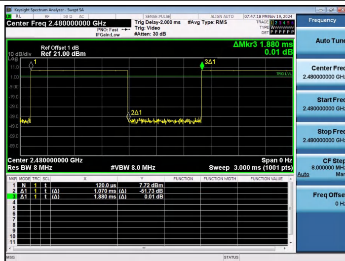
NTNV-BLE_2M-Ant1-2480
