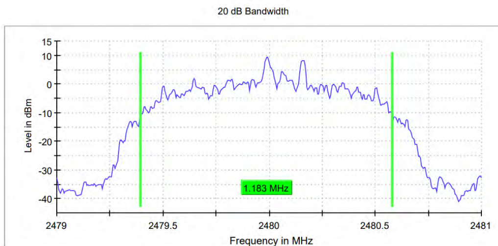
2DH5_Ant1_2480
