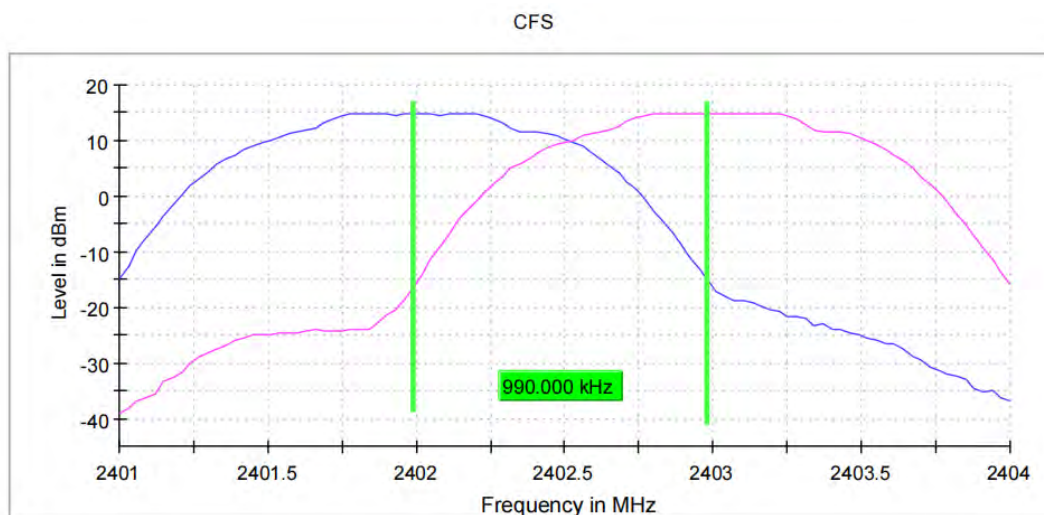
DH5_Ant1_Hop
