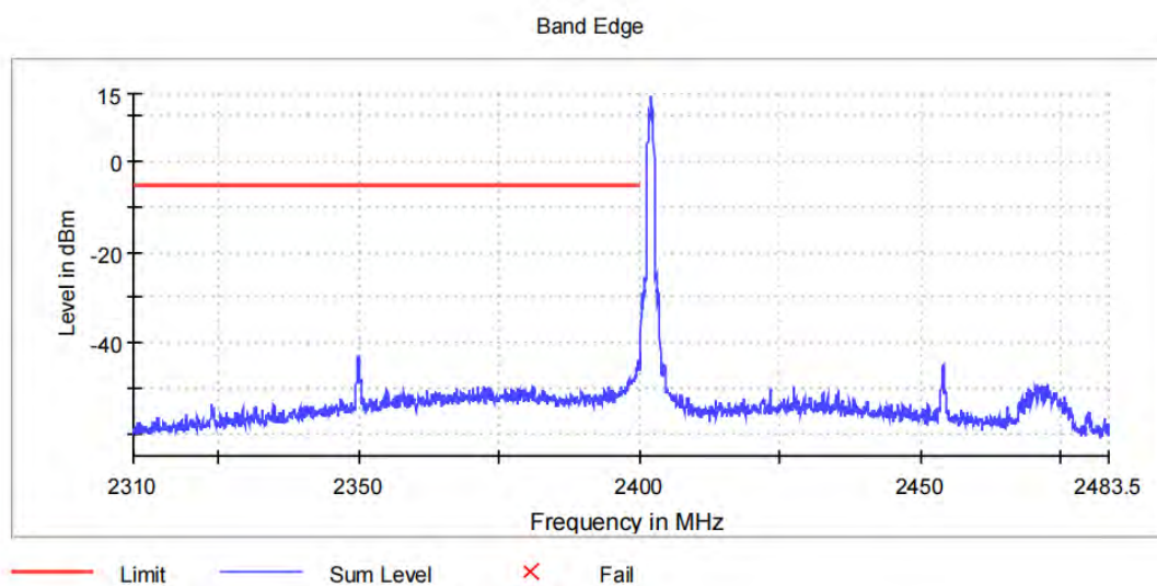
DH5_Ant1_Low_2402
