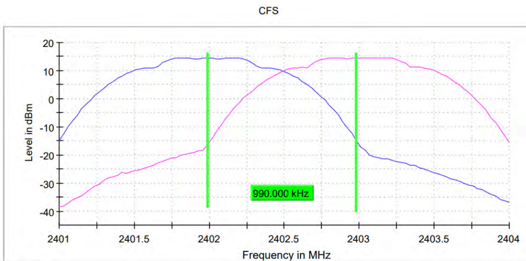
2DH5_Ant1_Hop
