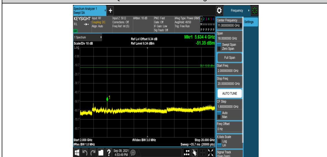
Band25-10MHz-QPSK-26365-1RB#0-Range5:2000~20000MHz
