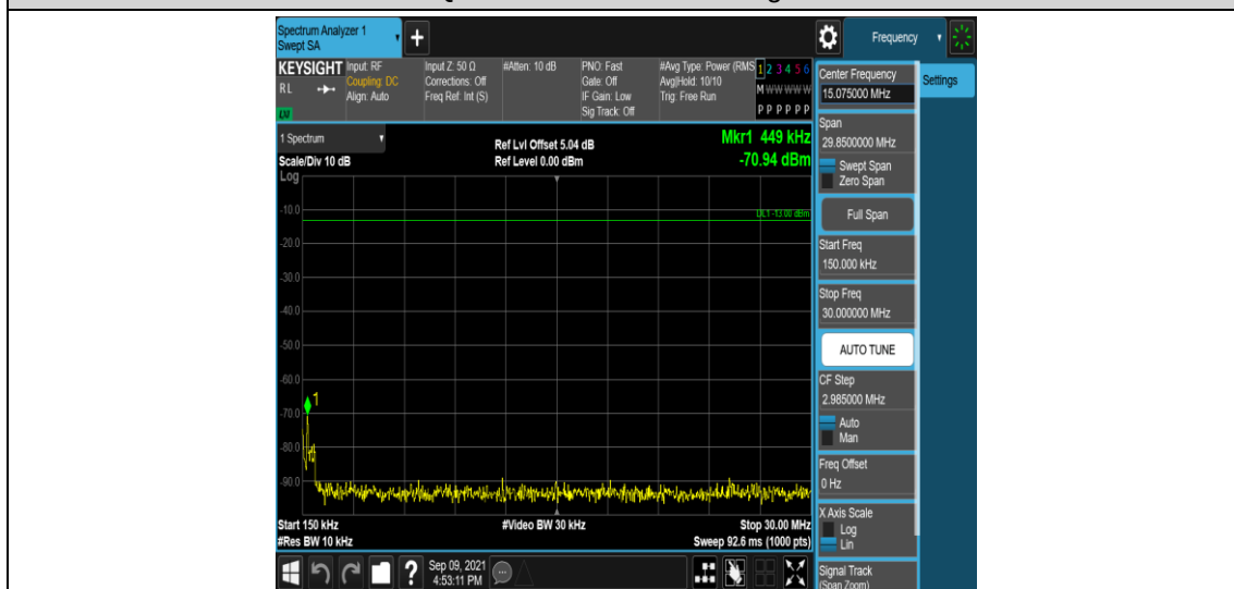
Band25-10MHz-QPSK-26365-1RB#0-Range2:0.15~30MHz
