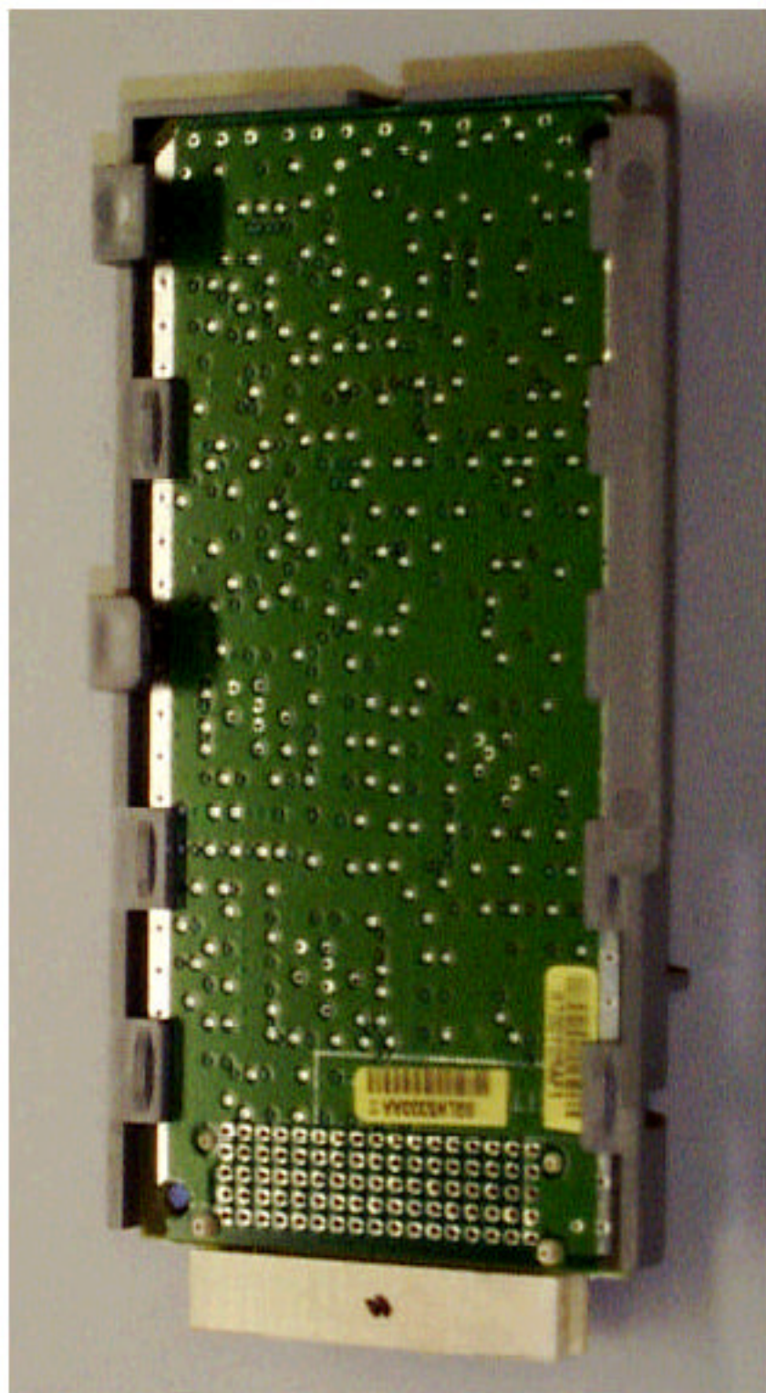
IHET5ZR1 SC4812ET 800 MHz CCD Back
