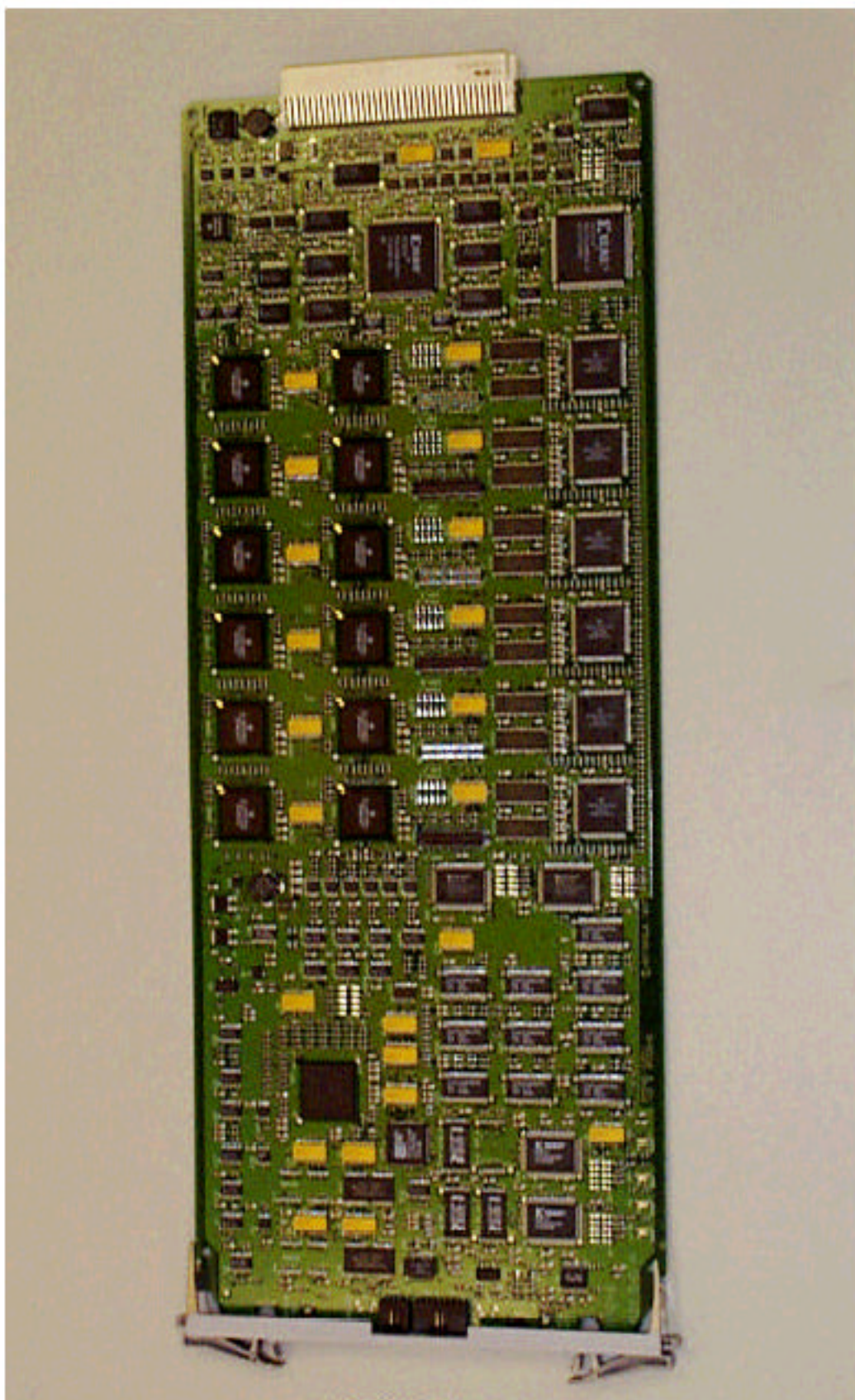
IHET5ZR1 SC4812ET 800 MHz MCC x 24E Front
