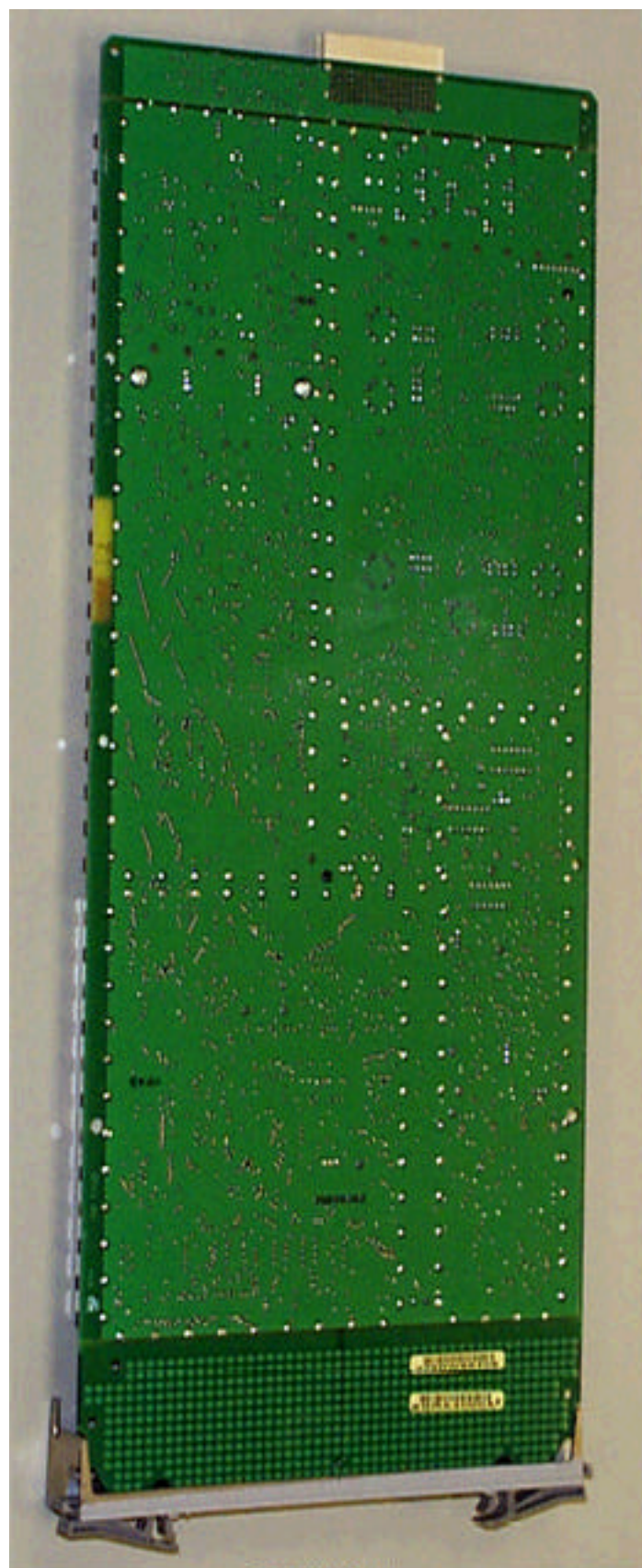
IHET5ZR1 SC4812ET 800 MHz LFR Back
