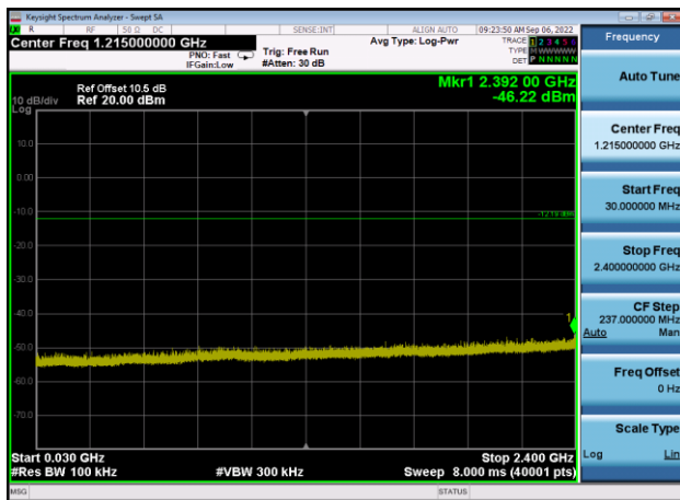
,Plot 3,30MHz~2400MHz-802.11g,2462MHz
