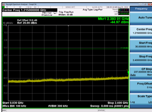
,Plot 3,30MHz~2400MHz-802.11g,2462MHz
