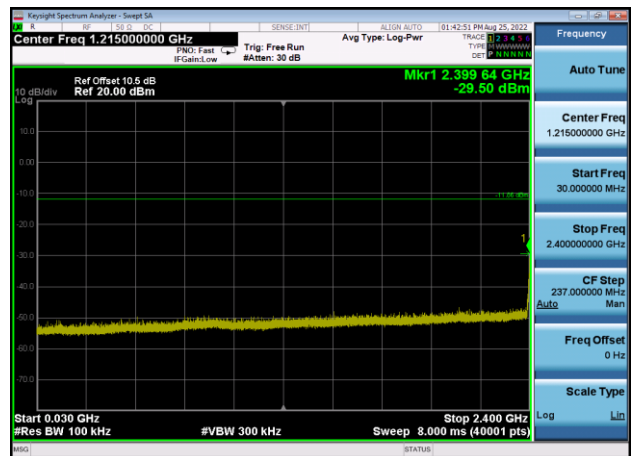
,Plot 3,30MHz~2400MHz-802.11g,2437MHz
