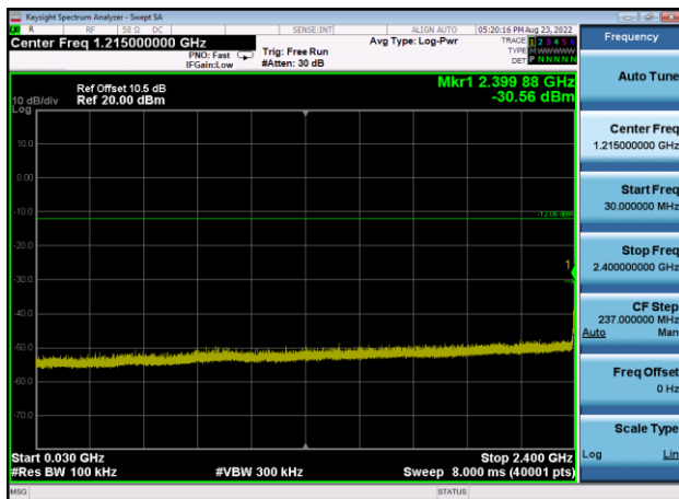
,Plot 3,30MHz~2400MHz-802.11g,2437MHz
