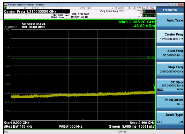
,Plot 3,30MHz~2400MHz-802.11g,2462MHz
