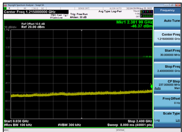
,Plot 3,30MHz~2400MHz-802.11g,2462MHz
