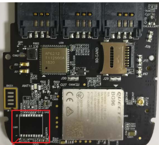
remove the GPS module
