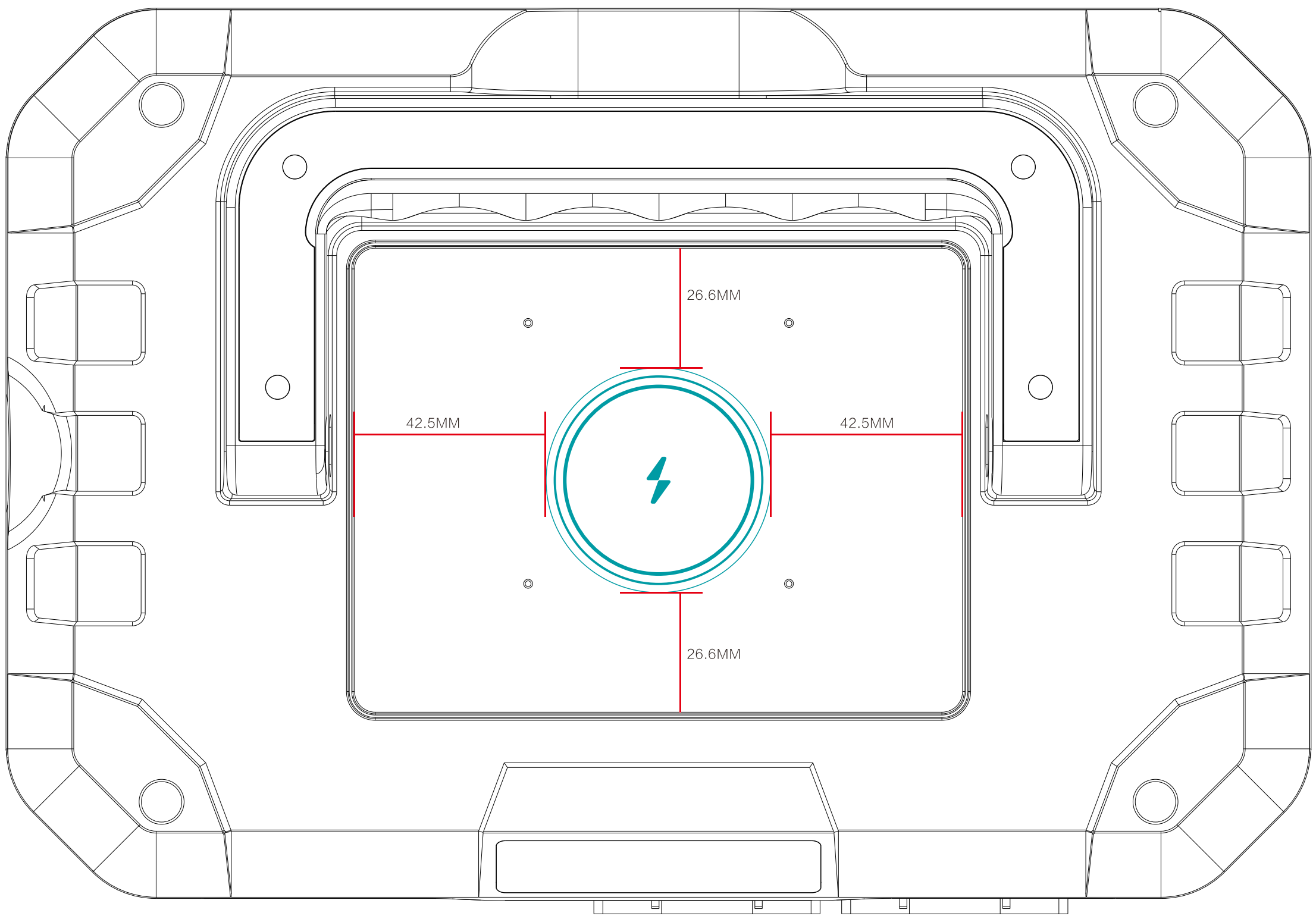
顶面
