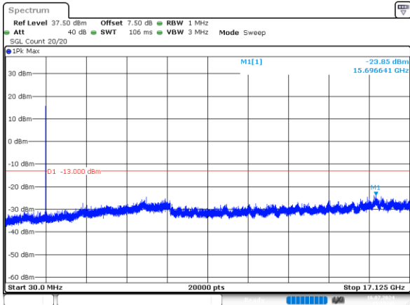
5MHz_Low_QPSK_25@0 -23.85dBm
