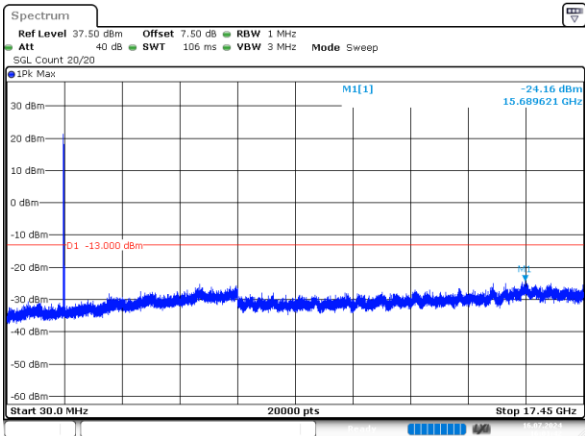
15MHz_Middle_QPSK_1@0 -24.16dBm
