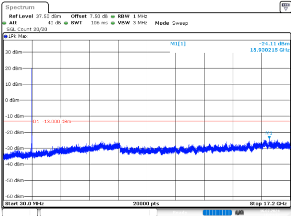
20MHz_Low_QPSK_1@0 -24.11dBm
