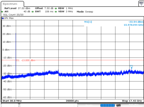
5MHz_Middle_QPSK_1@0 -23.94dBm
