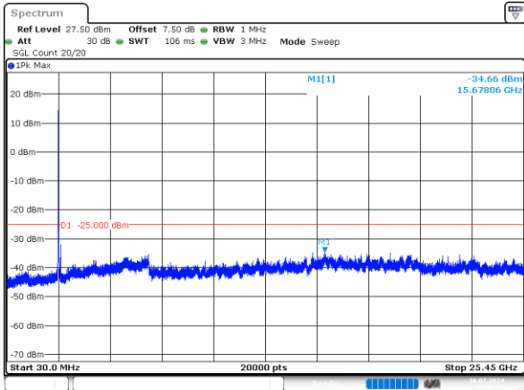
2_20MHz_Low_QPSK_100@0 -34.66dBm
