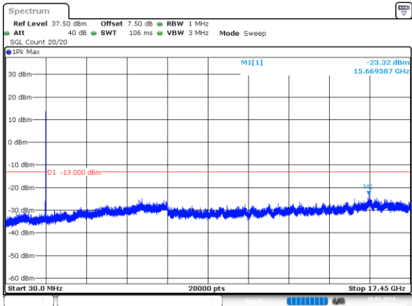
10MHz_Middle_QPSK_50@0 -23.32dBm
