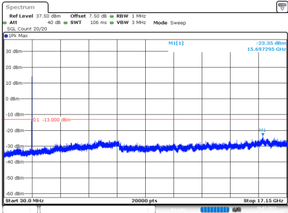
10MHz_Low_QPSK_50@0 -23.35dBm
