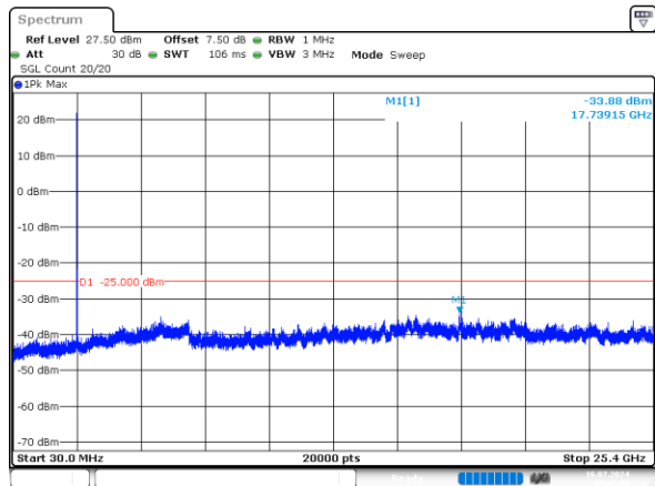
2_10MHz_Low_QPSK_1@0 -33.88dBm
