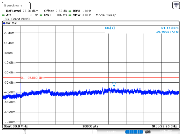
2_10MHz_Middle_QPSK_50@0 -34.44dBm
