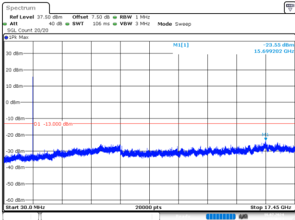
5MHz_Middle_QPSK_25@0 -23.55dBm
