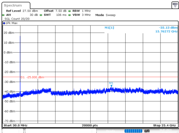
2_10MHz_Low_QPSK_50@0 -35.13dBm
