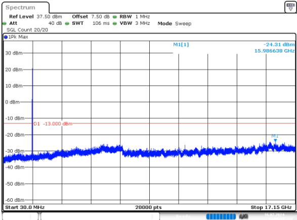
10MHz_Low_QPSK_1@0 -24.31dBm
