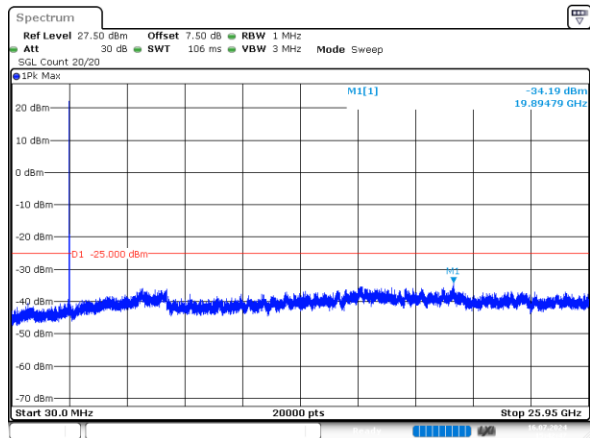
2_10MHz_Middle_QPSK_1@0 -34.19dBm
