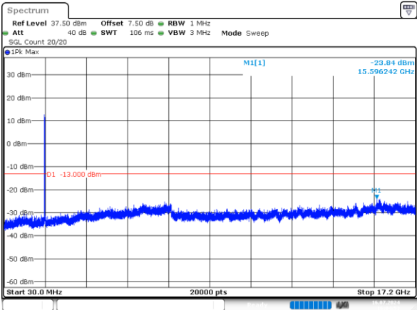
20MHz_Low_QPSK_100@0 -23.84dBm
